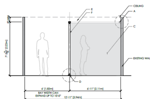
A2 SIDE ELEVATION SCALE: 3/16" = 1'-0"
