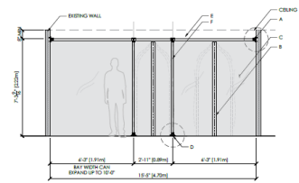
A1 FRONT ELEVATION SCALE: 3/16" = 1'-0"
